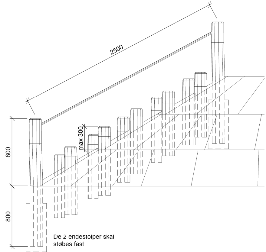
Sidebillede
