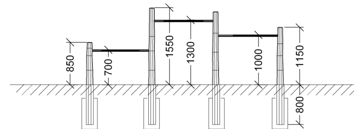
Sidebillede
