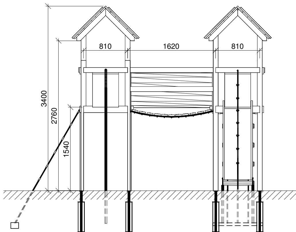
Stolpesko - brandmandsstang - støbebeslag skal støbes fast.
