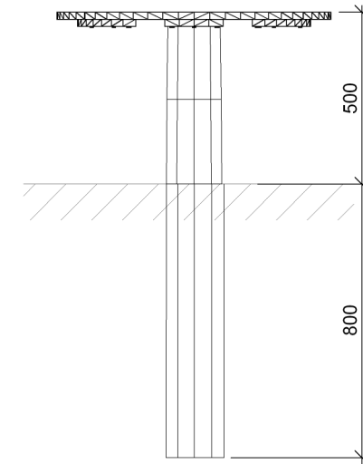
Sidebillede
